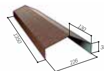
GAŚIOR DŁUGI CORONA AR130
