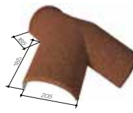
TRÓJNIK GAŚIORA 205 30-45°
