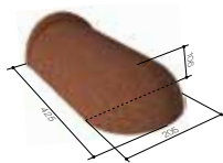
GAŚIOR POCZĄTKOWY 205
