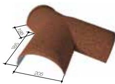
TRÓJNIK GAŚIORA 205 15-30°
